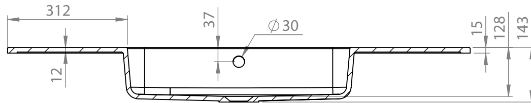
PRZEKRÓJ N-N SKALA 1 : 10
