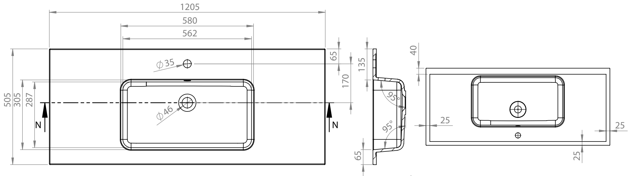
PRZEKRÓJ M-M SKALA 1 : 10
